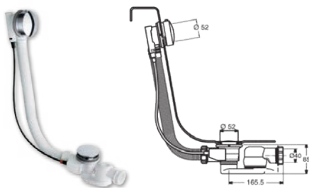
LUXE BADAFOER-/OVERLOOPCOMBINATIE chroom
