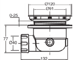
LUXE DOUCHEBAKAFVOER Ø 90 MM
